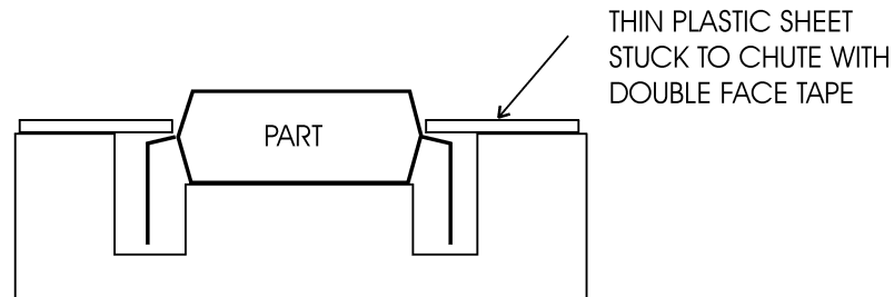
END ELEVATION
